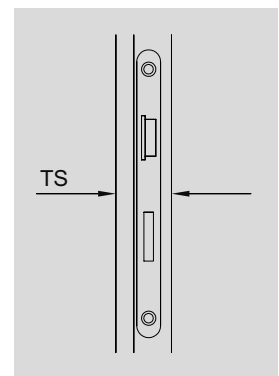
Standard-Türstärken
